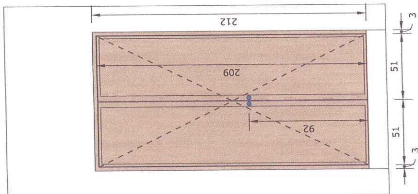
FRONTAL Esc.: 1/20
