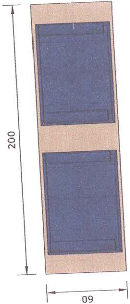
SUPERIOR Esc.: 1/20
