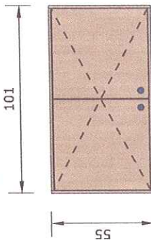
SUPERIOR Esc.: 1/20
