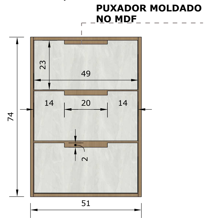
FRONTAL Esc.: 1/10
