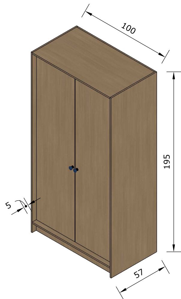
PERSPECTIVA 01 Esc.: 1/20
