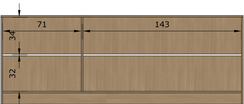
FRONTAL Esc.: 1/20
