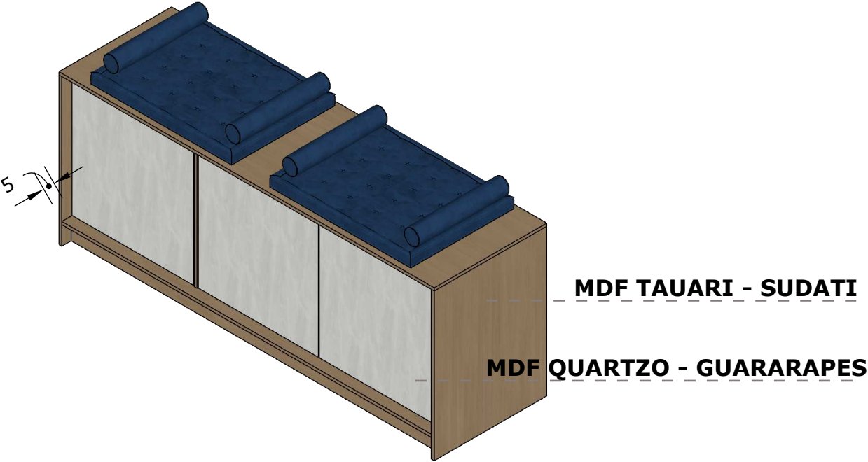
PERSPECTIVA 01 Esc.: 1/20
