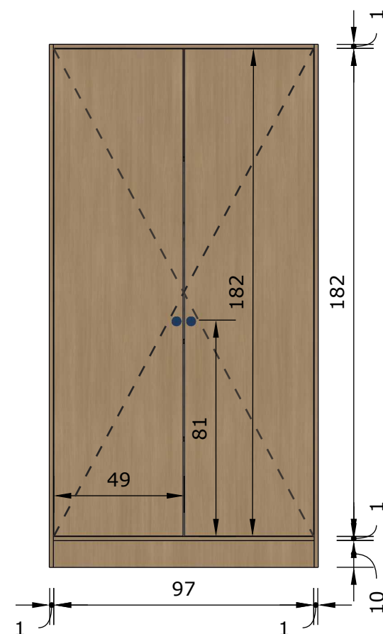
FRONTAL Esc.: 1/20
