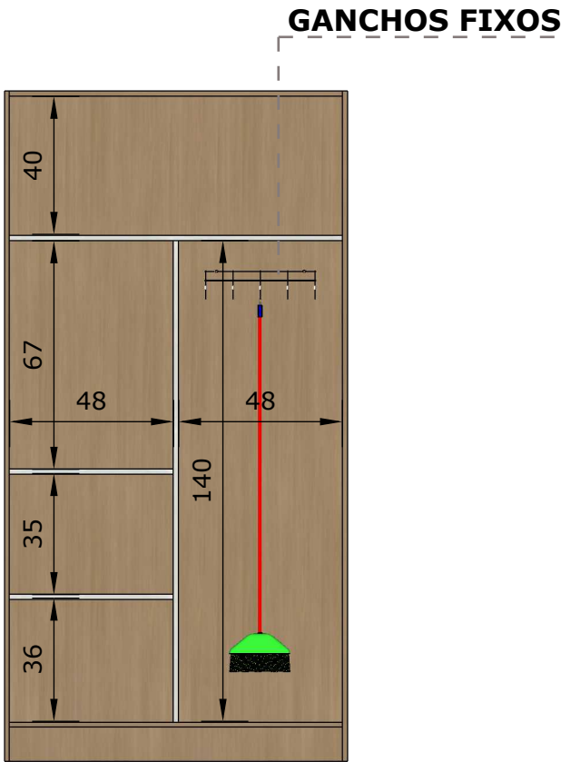
SUPERIOR Esc.: 1/20
