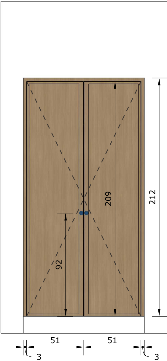
FRONTAL Esc.: 1/20
