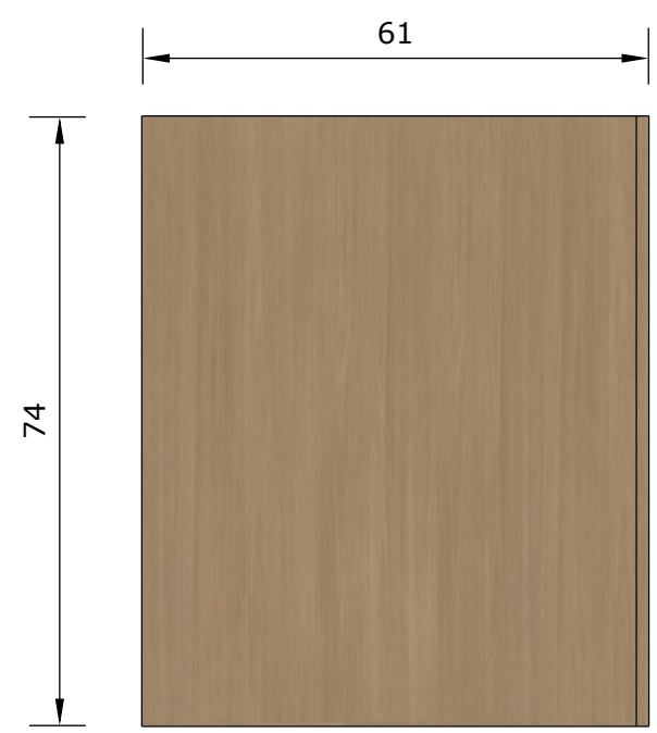
LATERAL Esc.: 1/10
