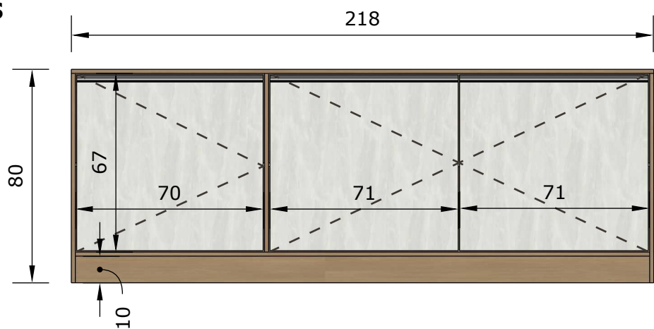
FRONTAL Esc.: 1/20
