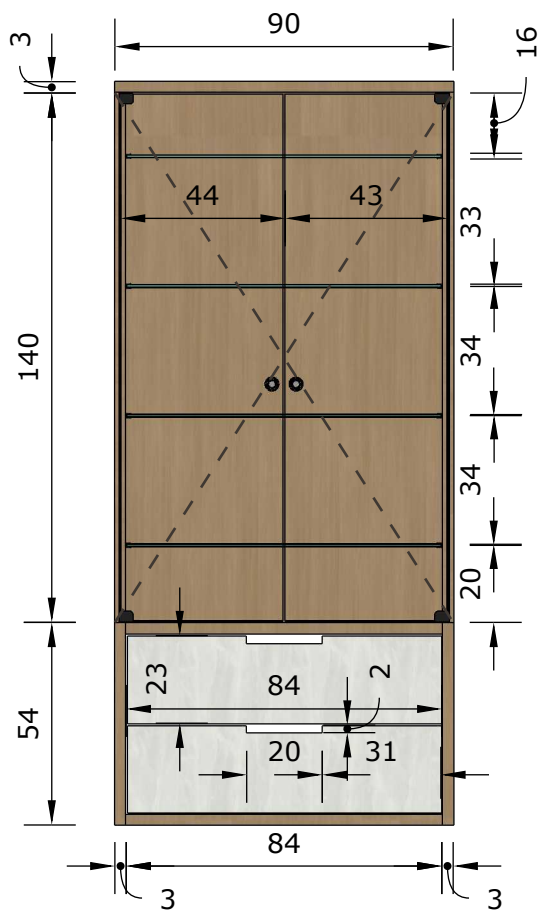
FRONTAL Esc.: 1/20
