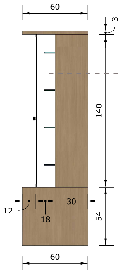
LATERAL Esc.: 1/20
