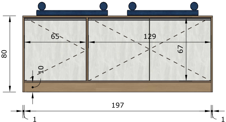
FRONTAL Esc.: 1/20
