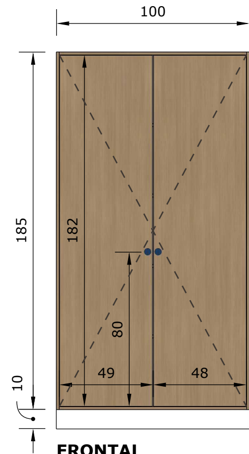
FRONTAL Esc.: 1/20
