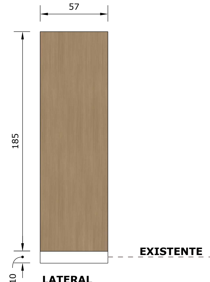
LATERAL Esc.: 1/20
