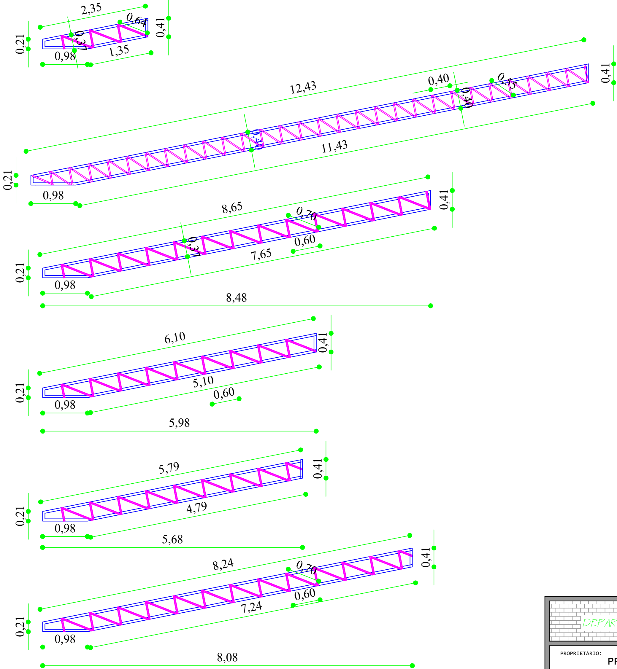
TESOURAS PARTE EXISTENTE - CONFERIR MEDIDAS IN-LOCO APÓS CONSTRUÇÃO DA PARTE PRÉ-FABRICADA
